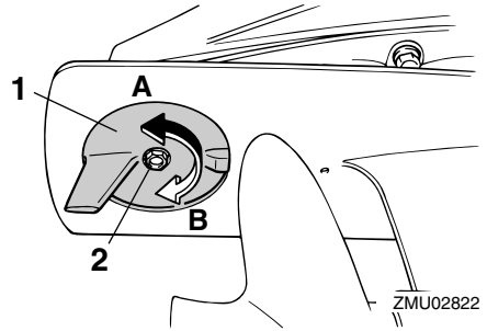
1. Trimmievä 2. Pultti
