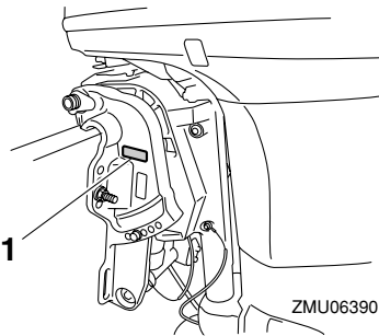
1. Placering av utombordsmotorns serienummer
