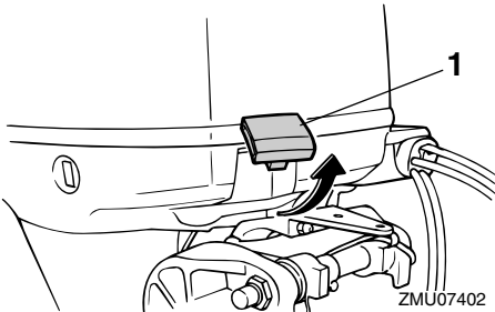
1. Kopan lukitusvipu/-vivut
