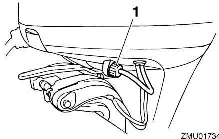
1. Gennemskylningsudstyr
