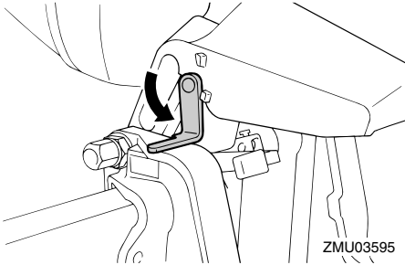
1. Spolanordning
