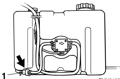
1. Oliefilter
