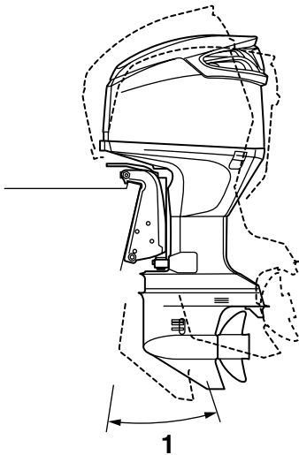
1. Trim arbejdsvinkel
