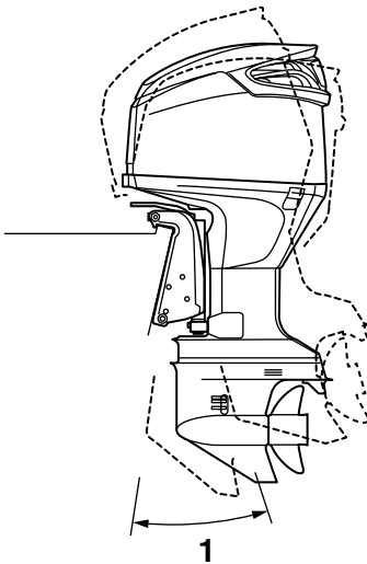
1. Trim arbejdsvinkel
