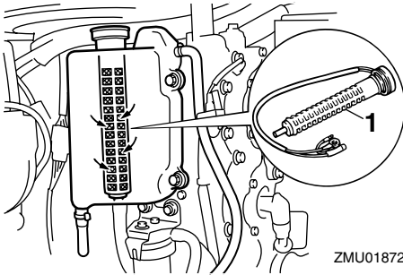
1. Oliefilter
