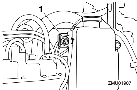
1. Varasäiliön täyttökytkin
