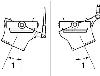
1 Γωνίες ακροφυσίου
