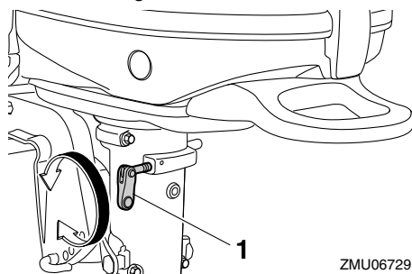
1. Justering af styringsfriktion
