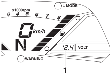
1 Voltmeter
