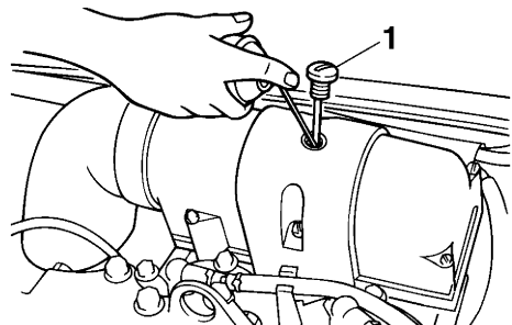
1 Καπάκι σιγαστήρα
