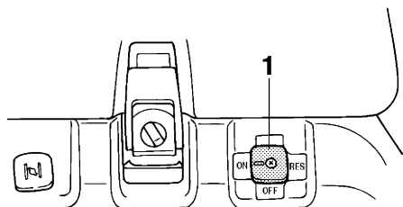
1 Διακόπτης καυσίμου
